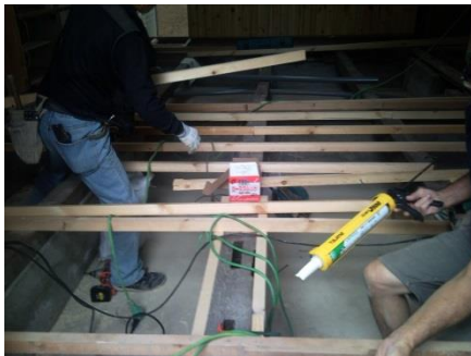
根太組み
